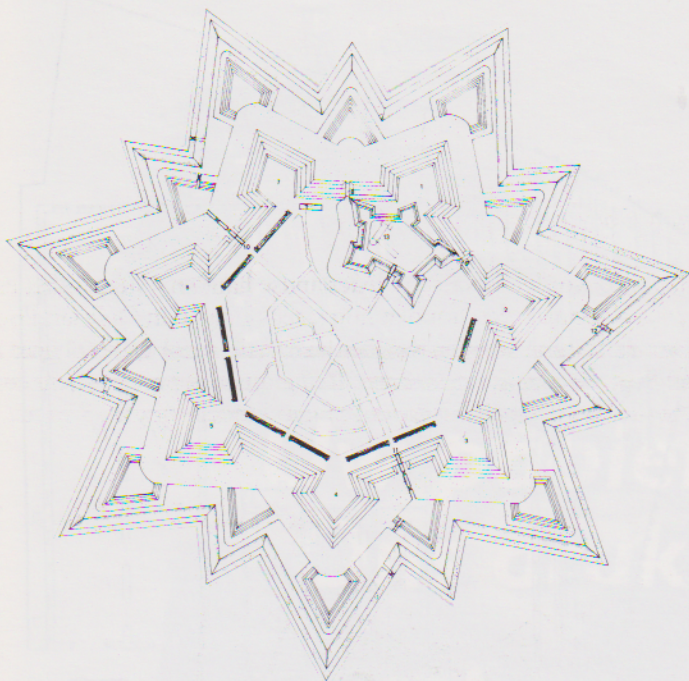
Tekening van de gereed gekomen vesting met duidelijk zichtbaar de kazernegebouwen. Het kasteel vormt een vesting in de vesting.
